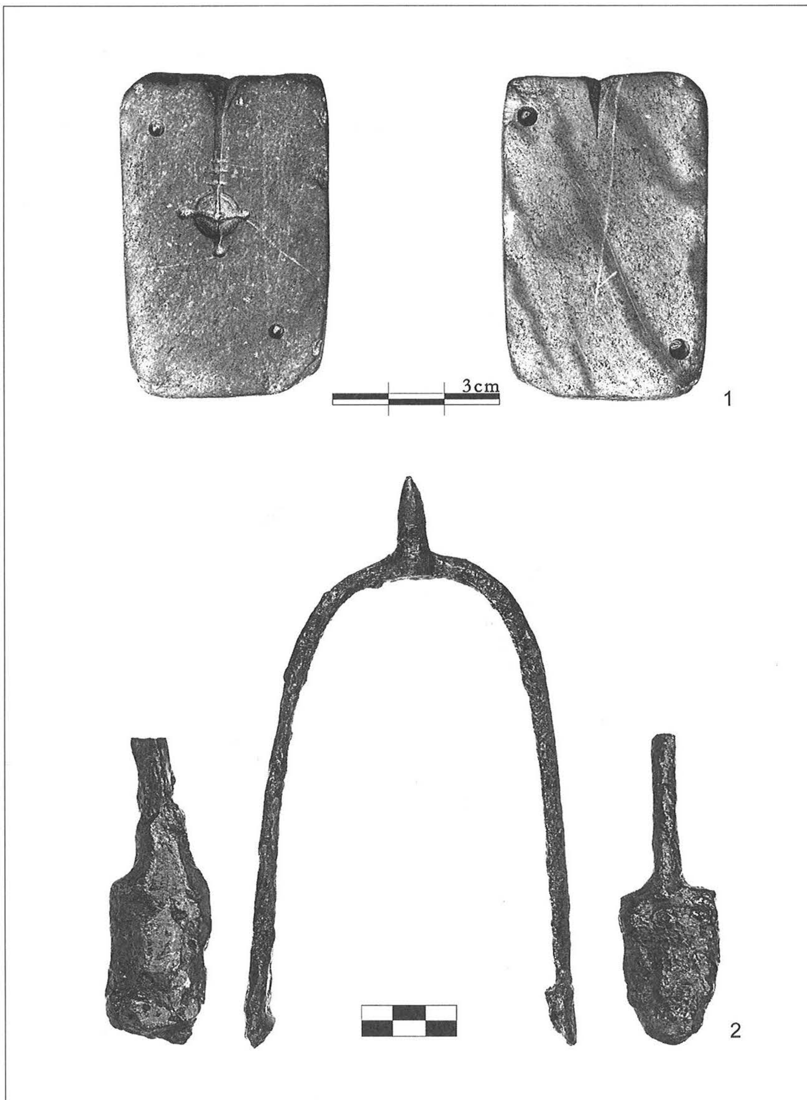
10. kép: Nagyrécse, Baráka-dűlő. Öntőforma, vassarkantyú. 1: 48. obj.; 2: 23. obj. Fig. 10: Nagyrécse, Baráka-dűlő. Mould, iron spur. 1: feature no. 48; 2: feature no. 23
