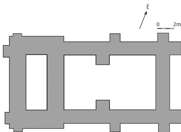
Iharos, Temető. A templom korai formájának alaprajza.
